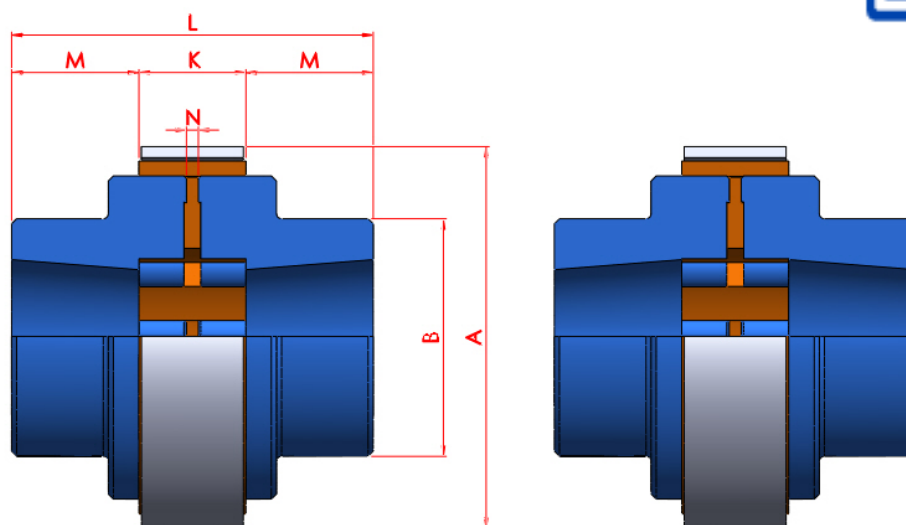
Acoflex para casquillo cónico. Serie AT
